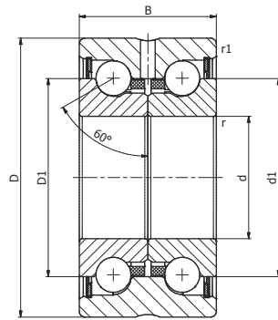
SEL/N...ZZ
