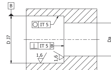
Housing PE
