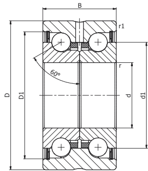
SEL/N...2RS / SEL/N...2RS.PE
