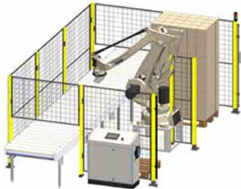
Robot antropomorfo
